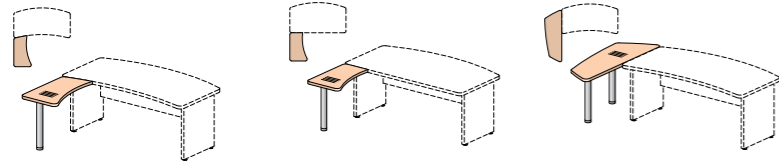
СП9-1(н1) 990x557x736 к столам СТ9-R18R, СТ9-18R, СТ9-R20R, СТ9-20R
